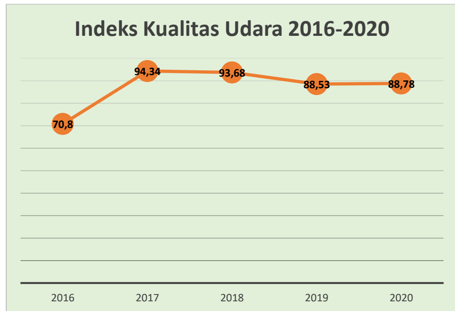
Gambar 2.3 Grafik Indeks Kualitas Udara
