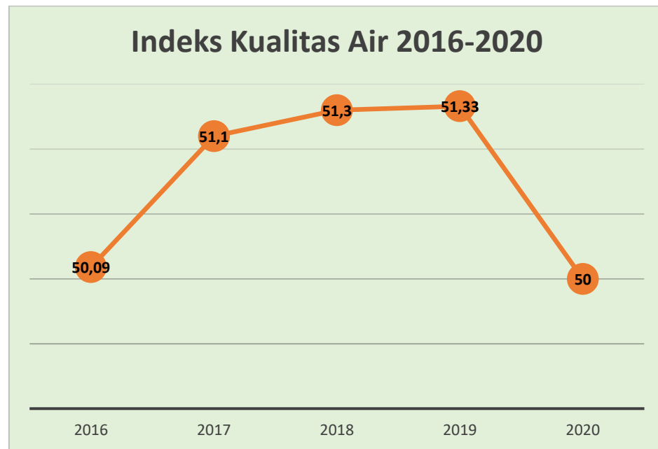
Gambar 2.2 Grafik Indeks Kualitas Air
