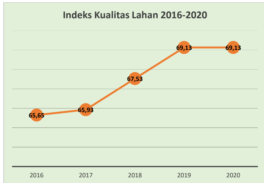
Gambar 2.4 Grafik Indeks Kualitas Lahan
