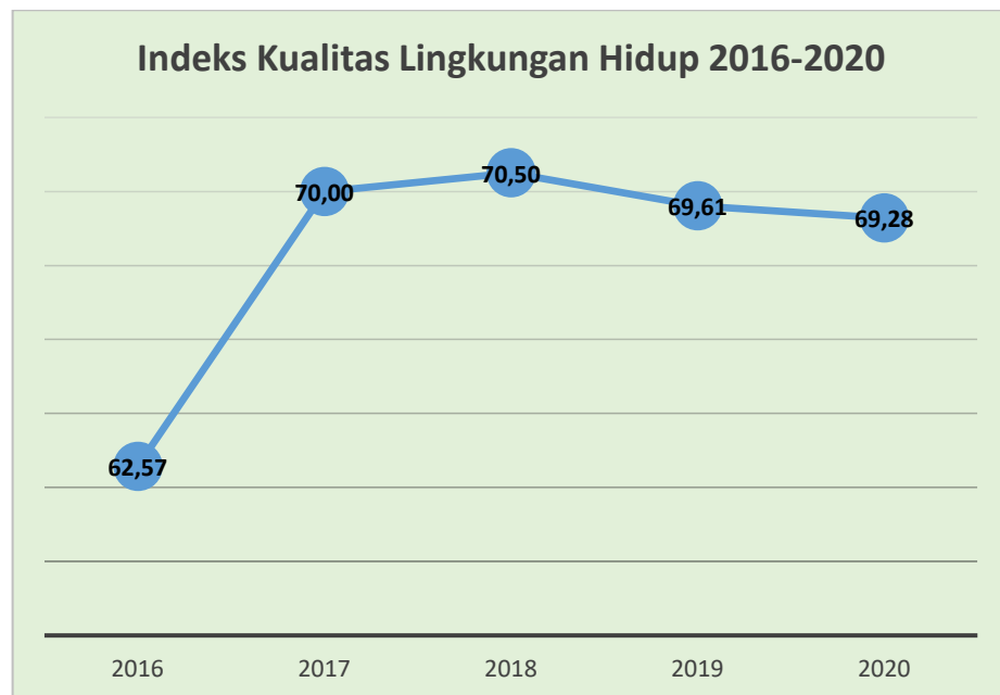
Gambar 2.5 Grafik Indeks Kualitas Lingkungan Hidup
