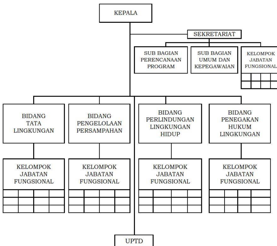
Gambar 2.1 Struktur Organisasi
